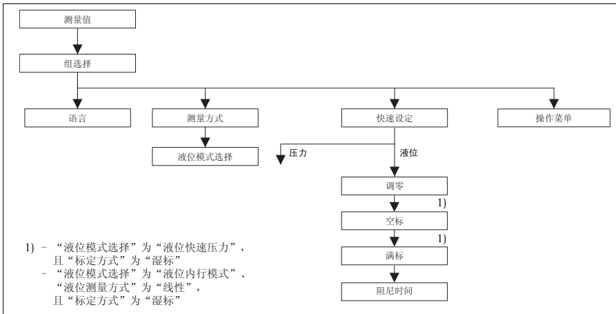
图 7: 液位测量方式的快速设定菜单
