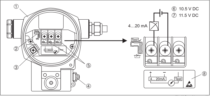
图 3: 4...20 mA HART 型仪表的电气连接示意图 → 请参考以下说明 带 Harting Han7D、M12 或 7/8" 插头的仪表, 请参考《操作手册》
