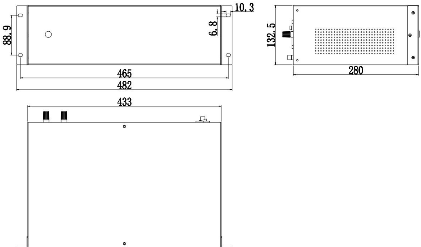
控制盒尺寸
