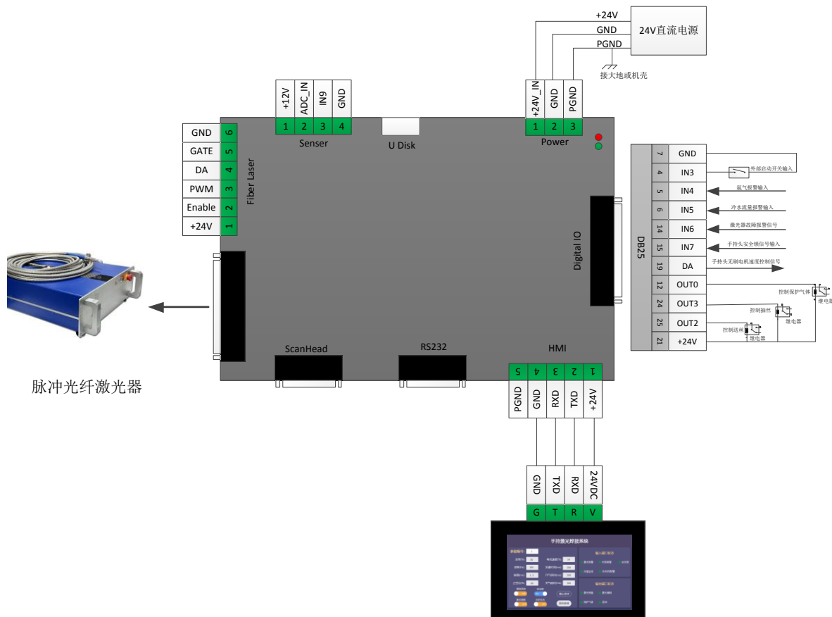
图 2.2 脉冲光纤激光器接线示意图
