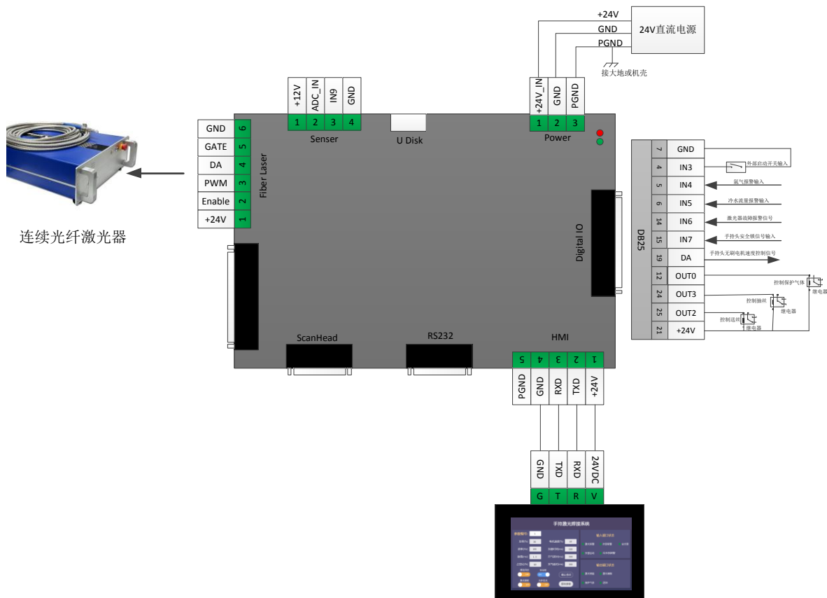
图 2.1 连续光纤激光器接线示意图
