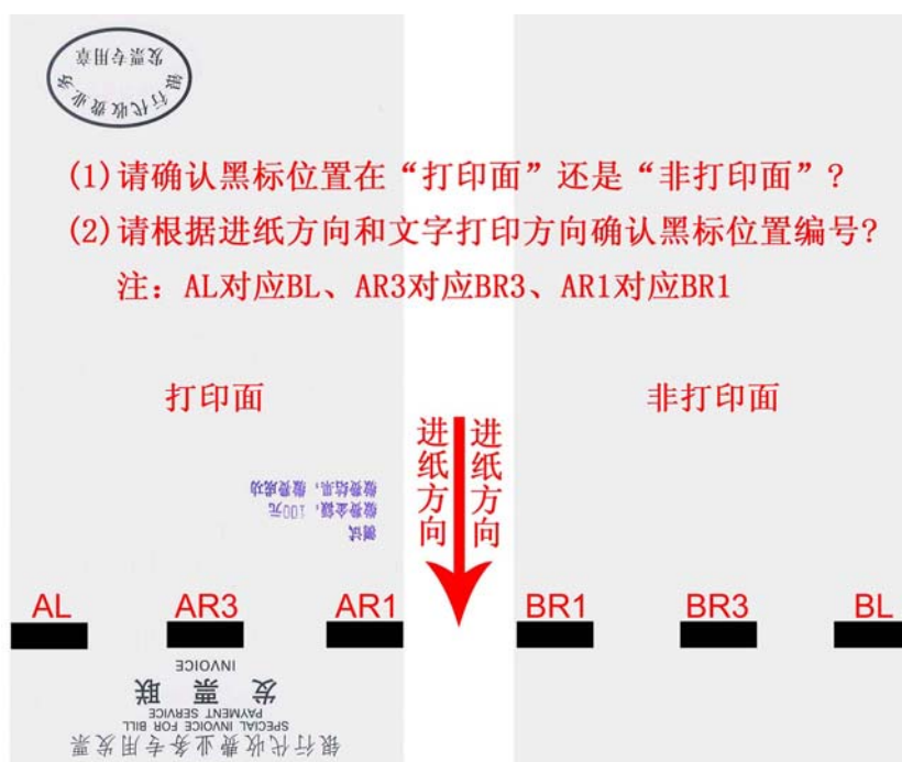
黑标探测位置图示
