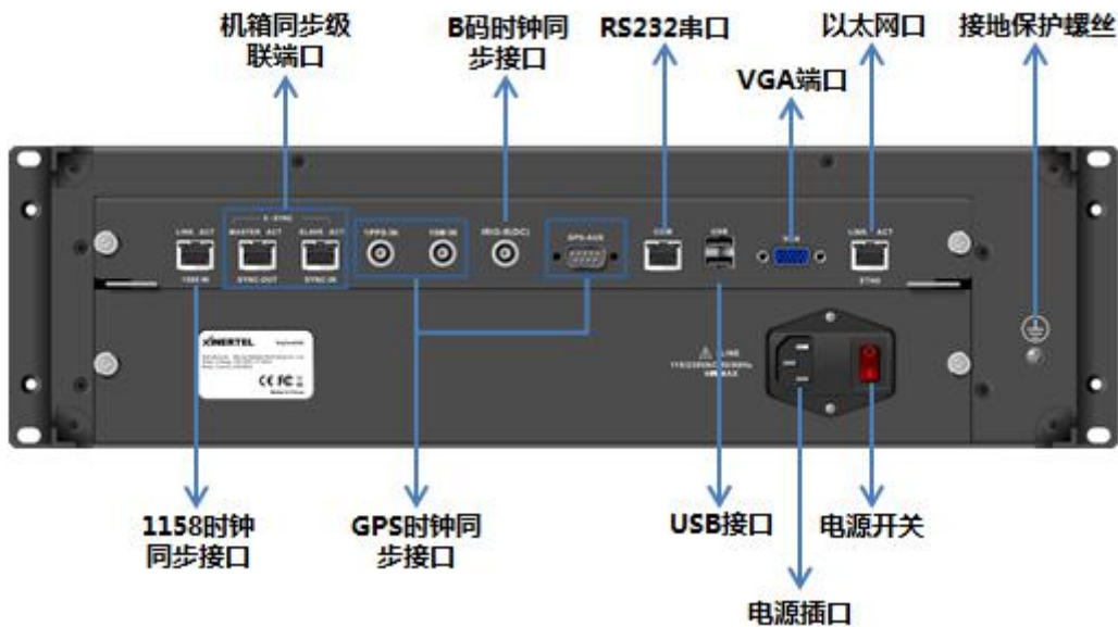
图 2 信而泰 BigTao6100 后面板示意图
