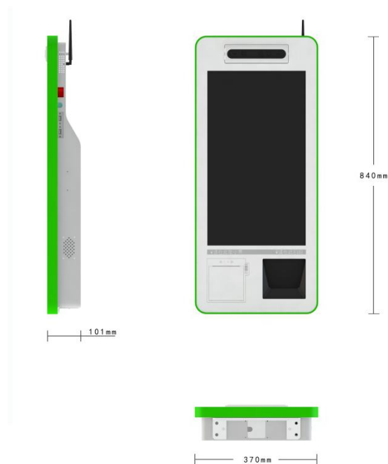
主机尺寸图
