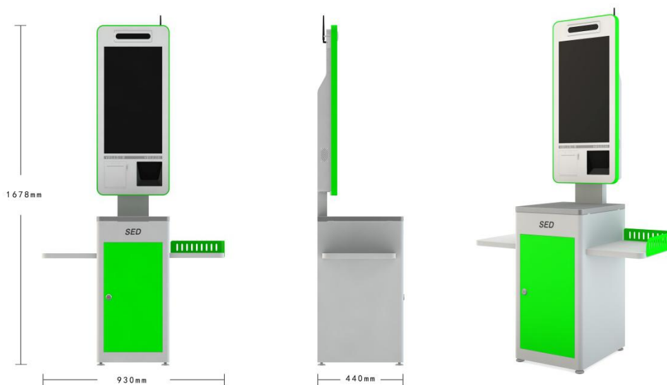
柜式支架版本尺寸图
