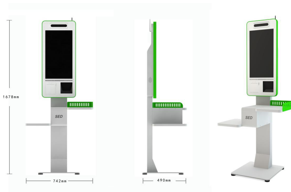
立式支架版本尺寸图
