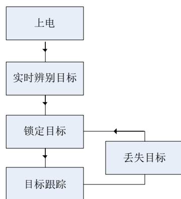
图 3 可见光探测器工作流程图
