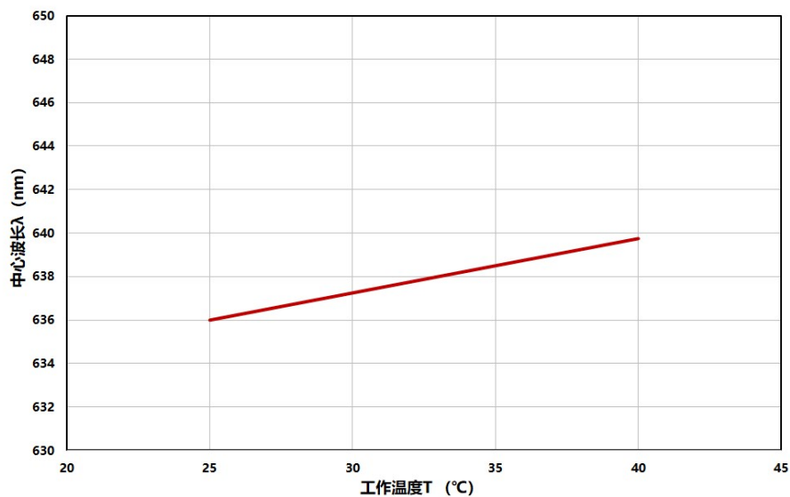
HGLD-635TO3.3-ZSP-5mW 各温度下中心波长
