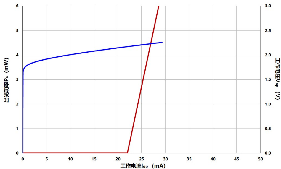
HGLD-635TO3.3-ZSP-5mW PIV 测试曲线
