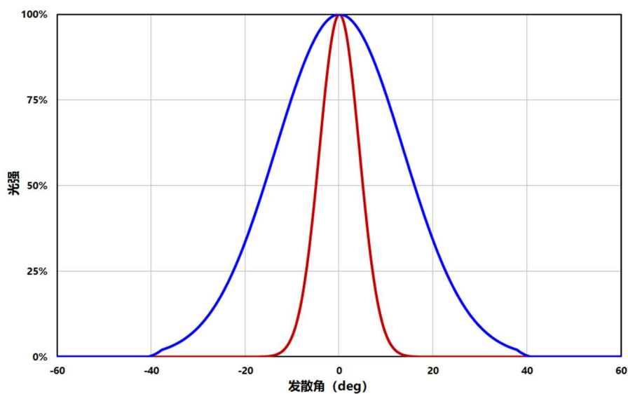
HGLD-635TO3.3-ZSP-5mW 远场光强分布
