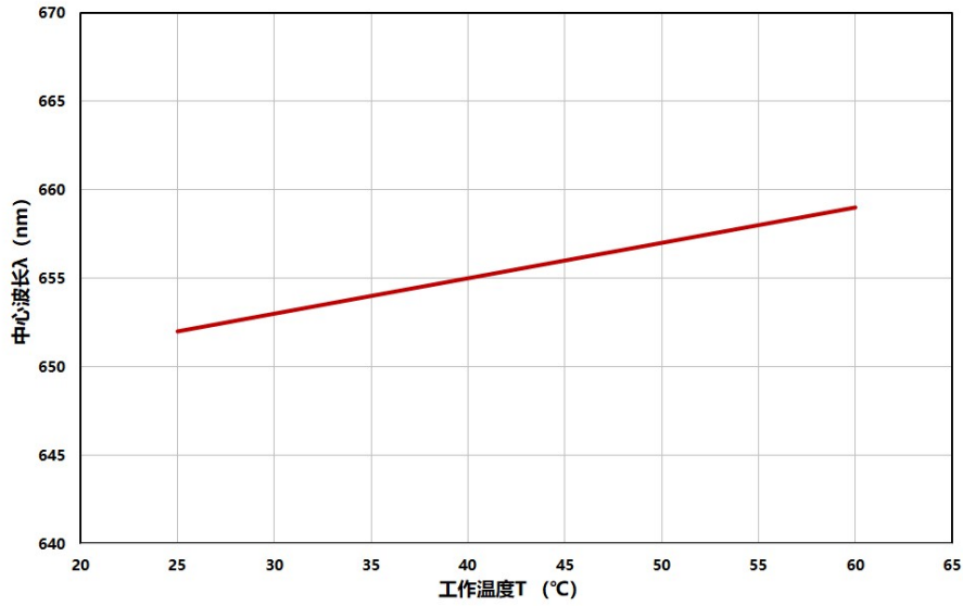
HGLD-650TO3.3-ZP-5mW 各温度下中心波长
