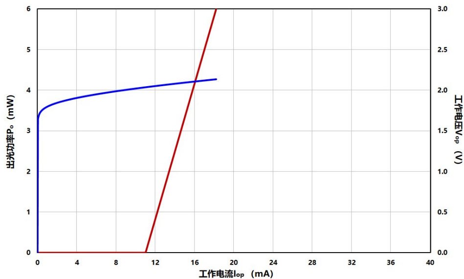
HGLD-650TO3.3-ZP-5mW PIV 测试曲线
