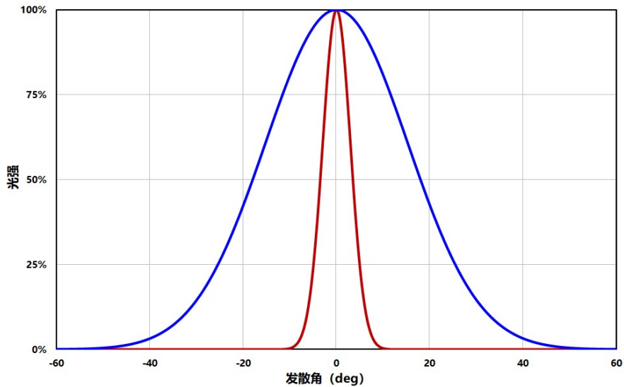
HGLD-650TO3.3-ZP-5mW 远场光强分布
