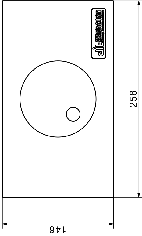
仰视图
