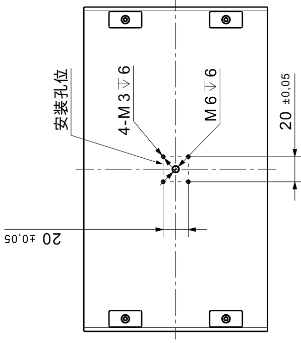
后视图
