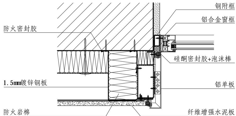
① 窗口横剖
