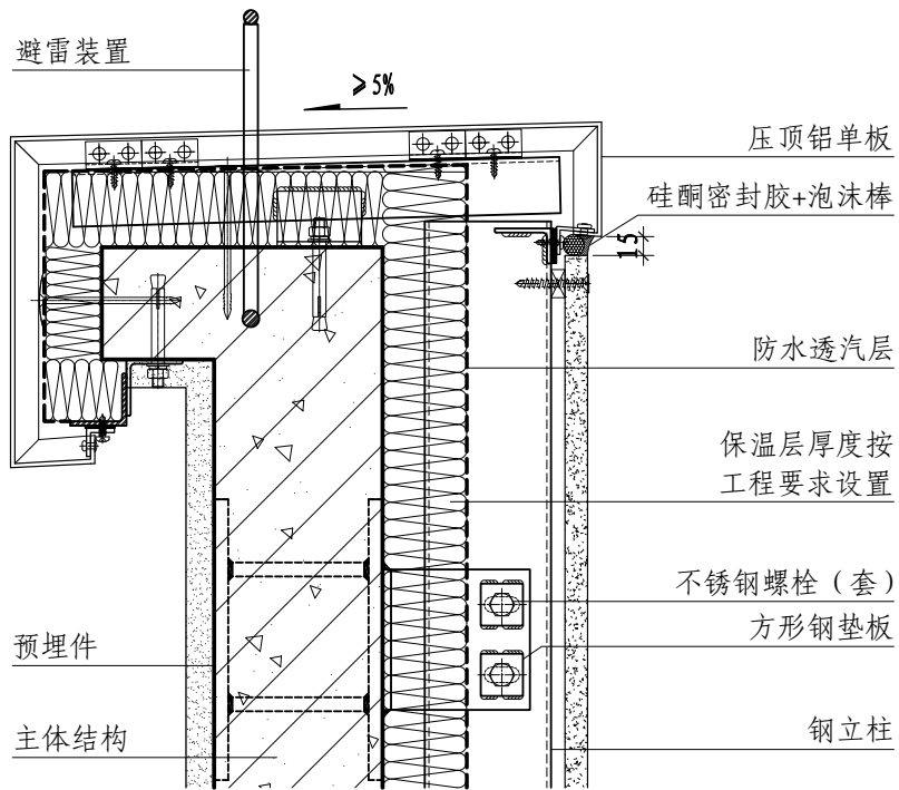
② 女儿墙部位
