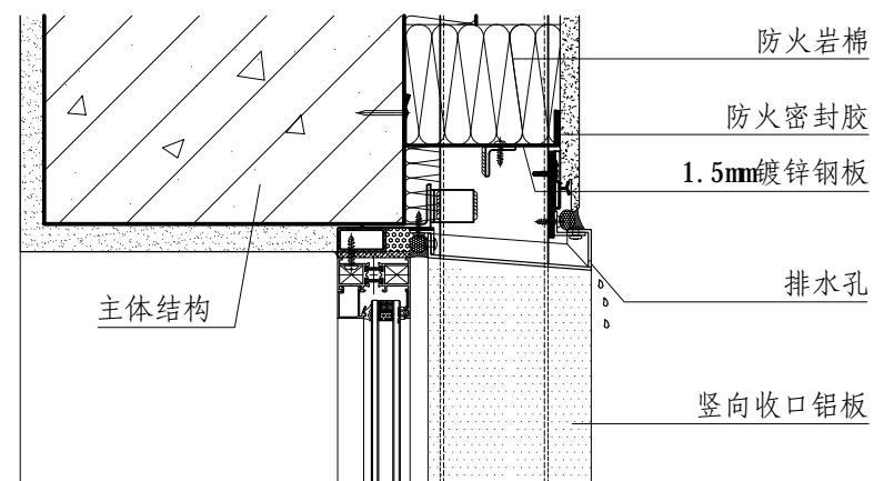
③ 窗上口
