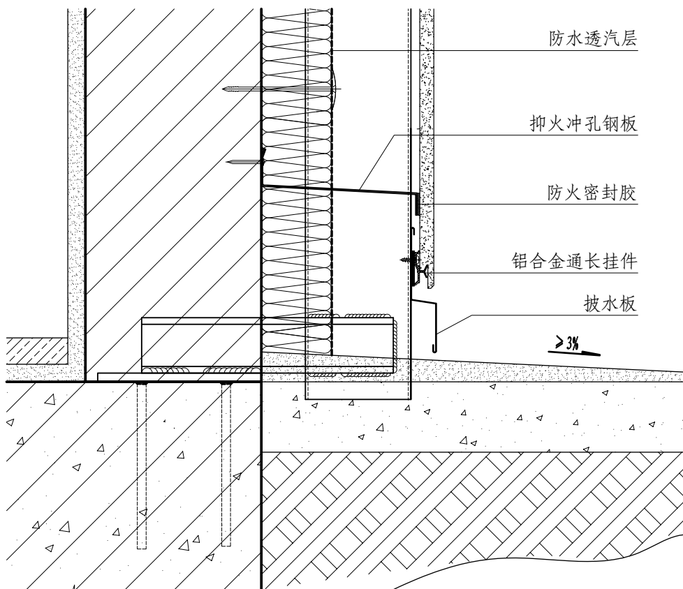
① 地面交接部位
