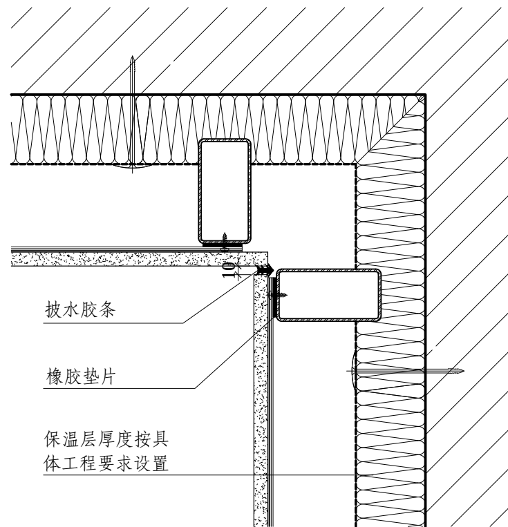
② 90° 阴角
