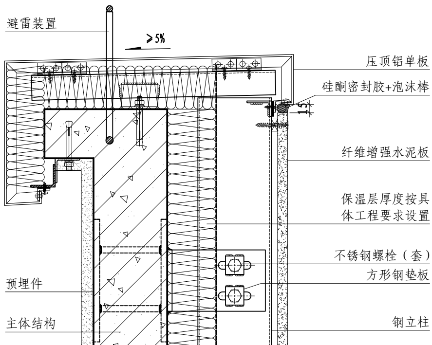
② 女儿墙部位
