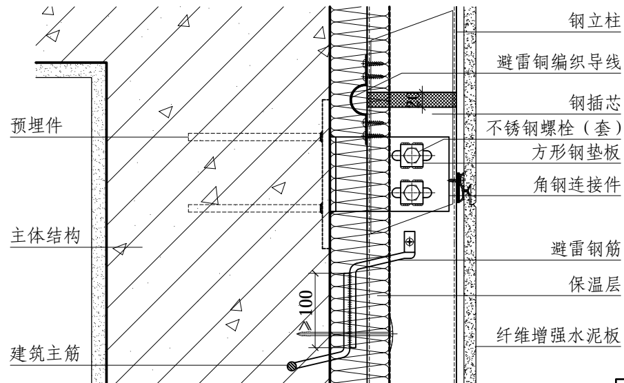
④ 层间防雷
