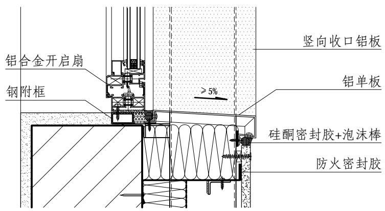
② 窗下口
