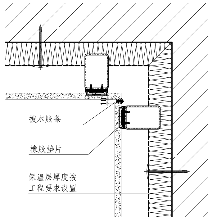
② 90° 阴角
