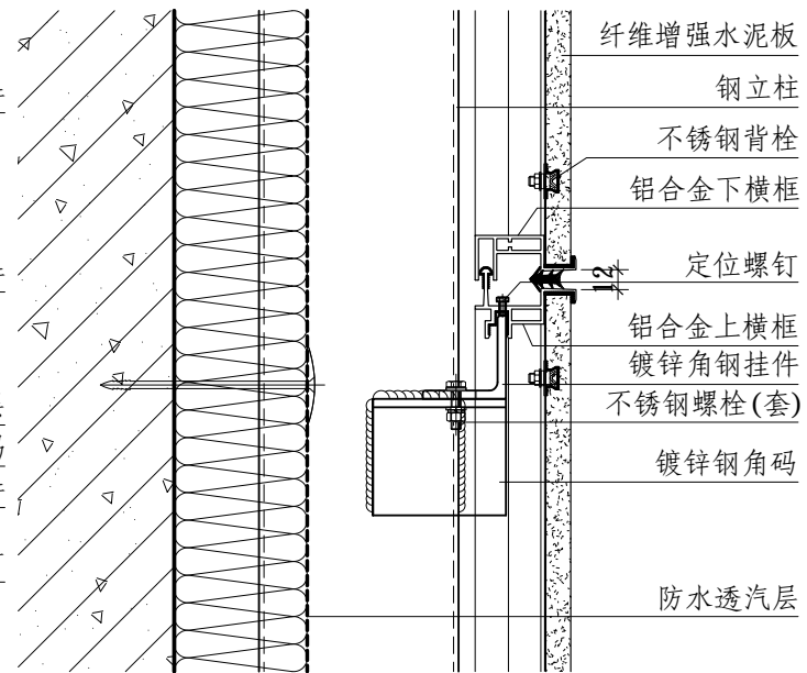
② 竖剖
