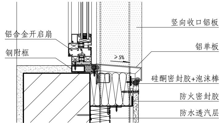
② 窗下口
