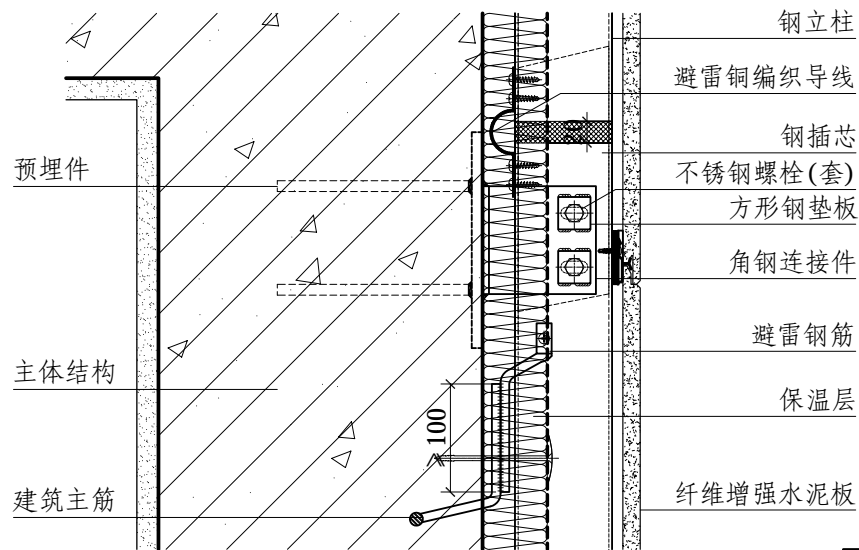
④ 层间防雷
