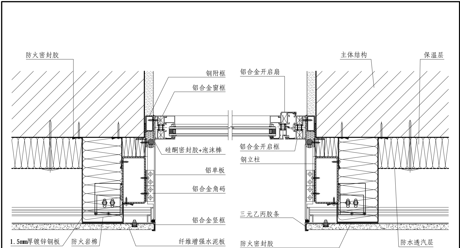
① 窗口横剖
