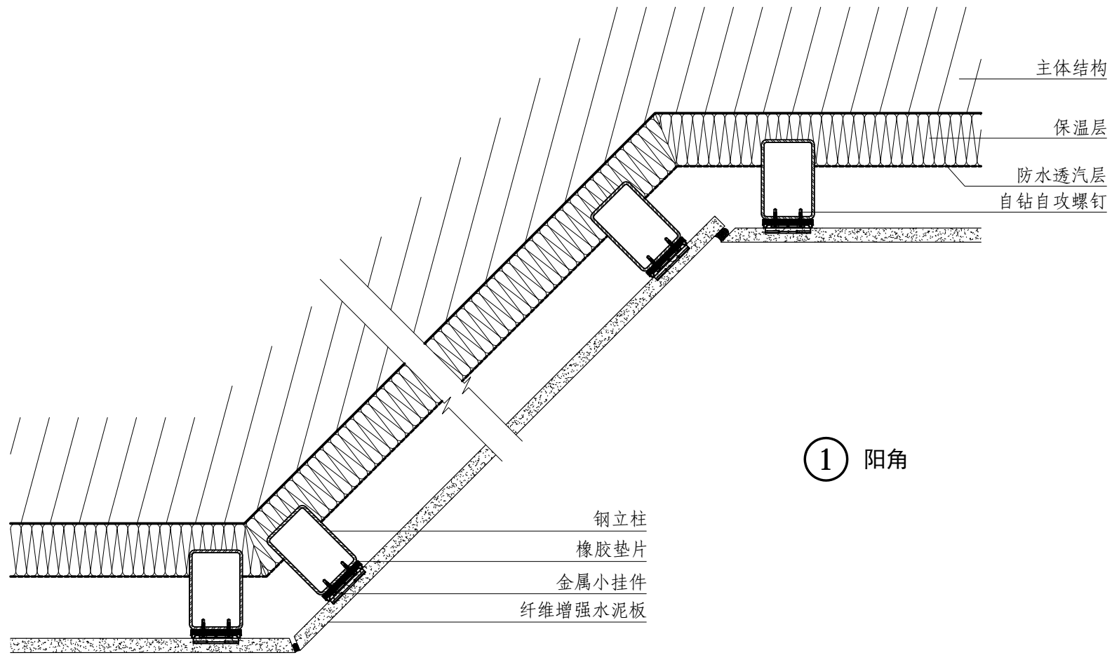
① 阳角
