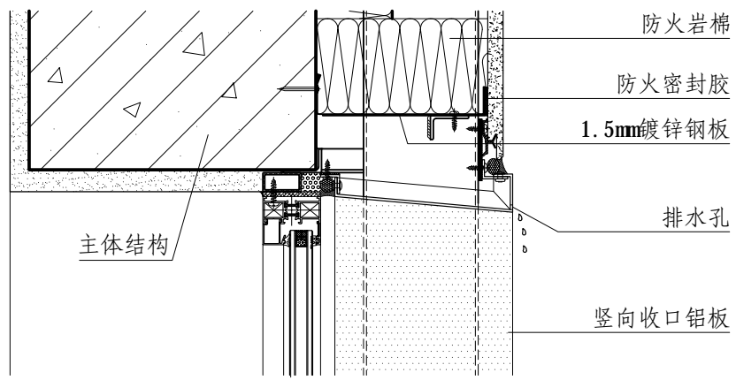
③ 窗上口
