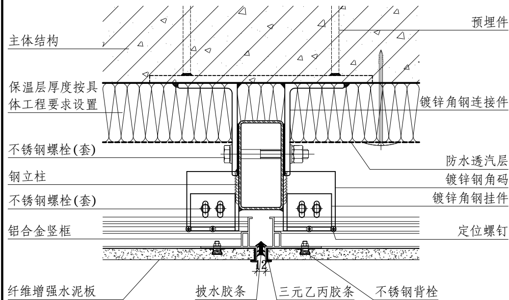
① 横剖
