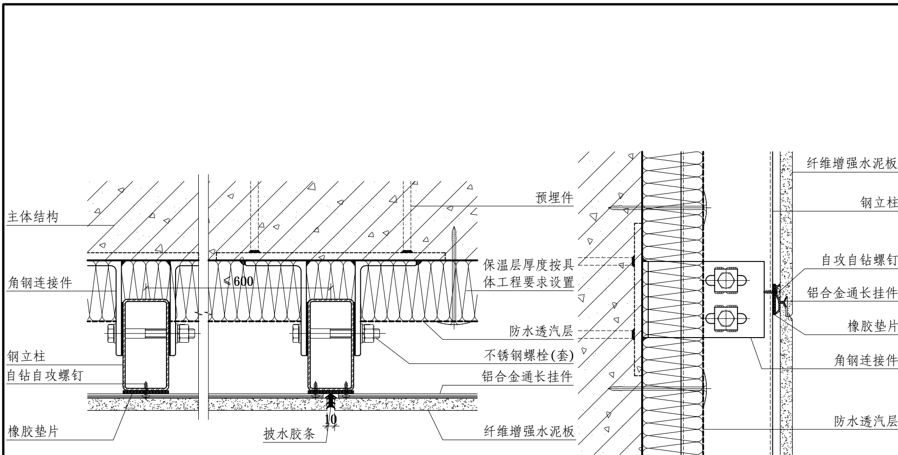
① 横剖
