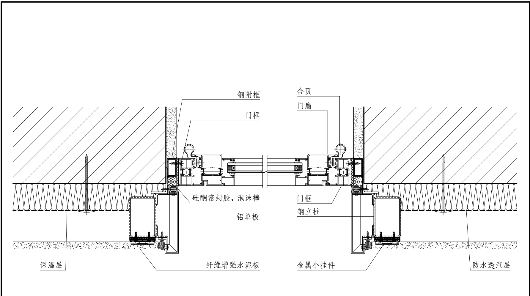
① 横剖
