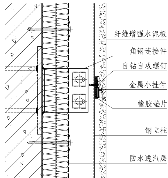
② 竖剖
