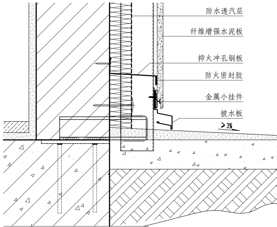
① 地面交接部位
