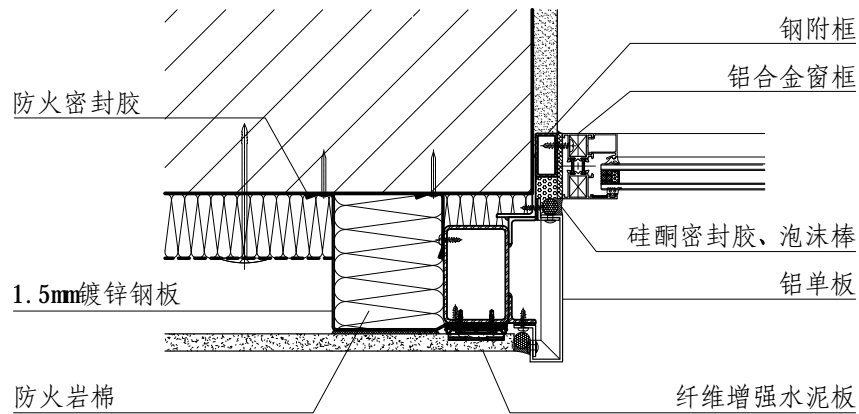
① 窗口横剖
