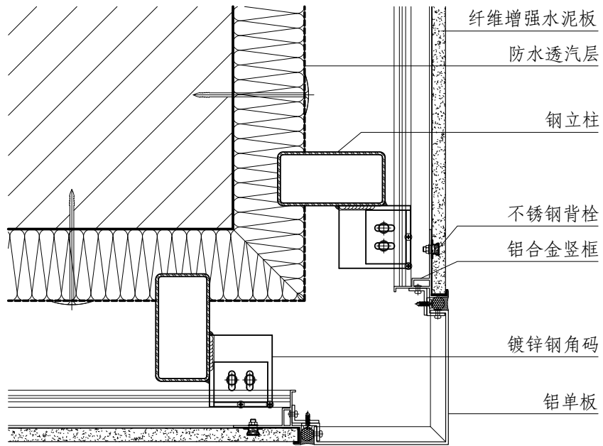
① 90° 阳角
