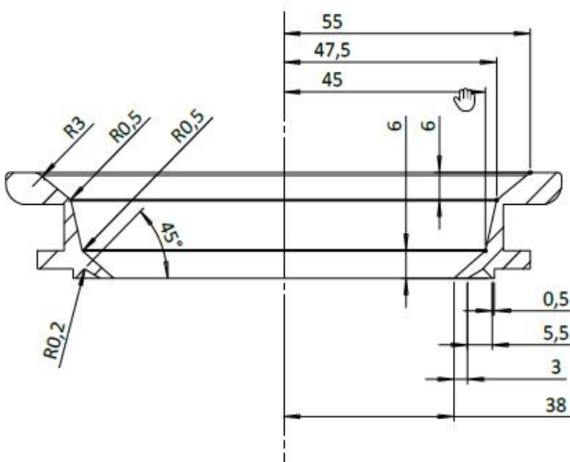
COUPE A-A
